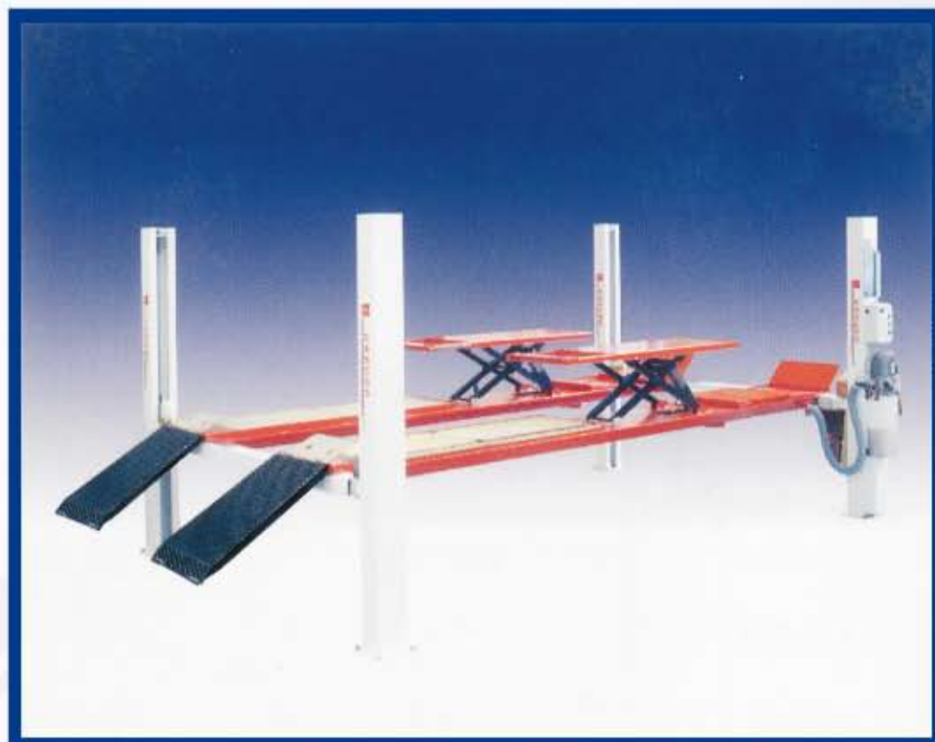
ELEVADOR DE 4 COLUMNAS CON DOBLE ELEVACIÓN
